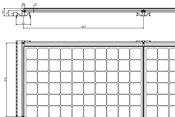
Technische Zeichnung 60-zellig
