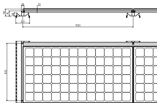
Technische Zeichnung 72-zellig
